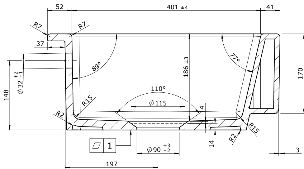
Corte A-A
